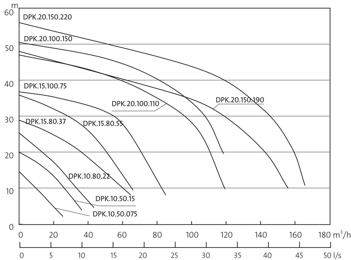
DPK性能曲线 (50Hz)
