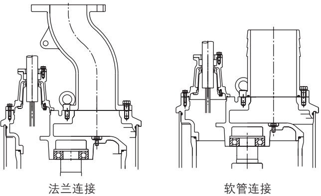
图2. DWK出口连接方式
