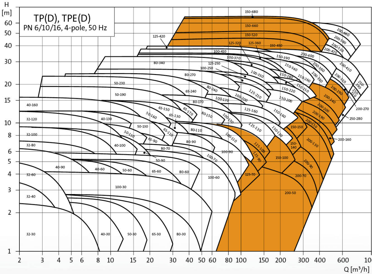
TP/TPE 50Hz 性能曲线和范围扩展图
