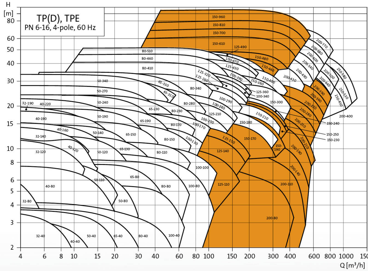
TP/TPE 60Hz 性能曲线和范围扩展图
